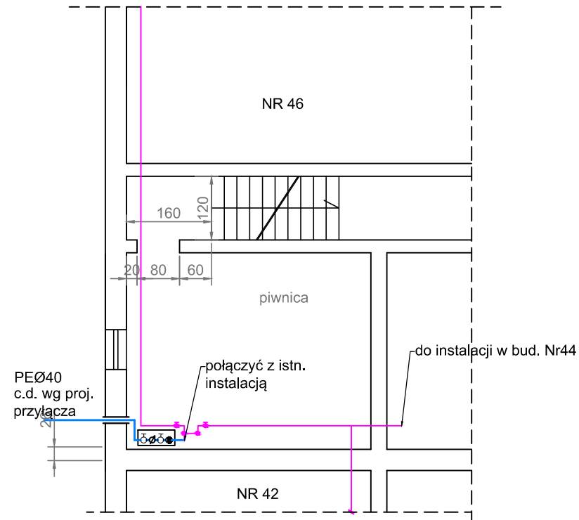
konsola wodomierzowa
